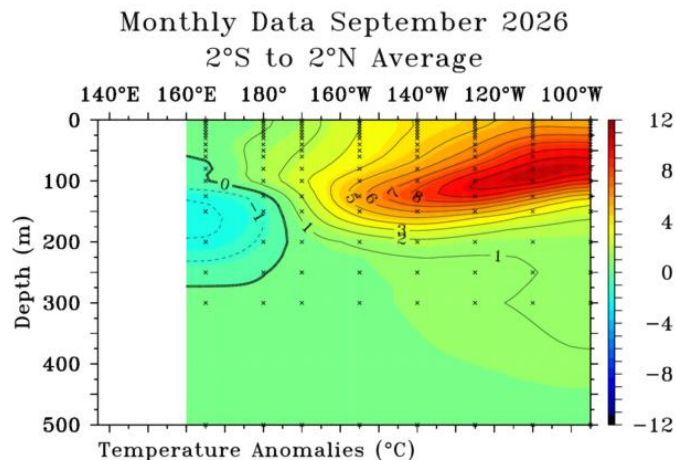
Figura 4 – Corte profundidad vs. longitud de la anomalía de temperatura del agua del mar en el Pacífico ecuatorial, correspondiente al promedio mensual de septiembre (izquierda) y pentádico que termina el 27 de septiembre (derecha). Fuente: Pacific Maritime Environmental Laboratory (PMEL)-NOAA
