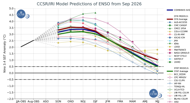
Figura 11 – Pronóstico de anomalías de TSM en la región Niño 3.4. Fuente: IRI.
