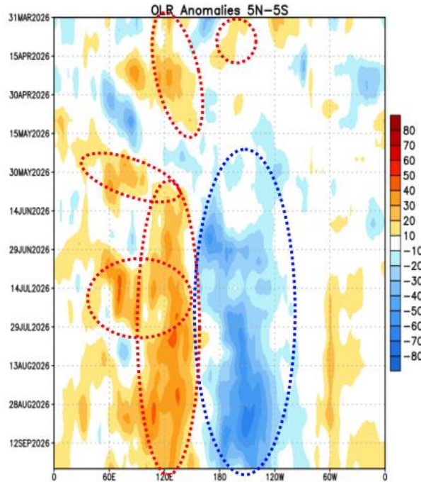
Figura 7 – Anomalías de radiación de onda larga saliente (OLR) promedio en la región 5°S-5°N, del 31 de marzo al 28 de septiembre de 2026 - Fuente: Climate Prediction Center (CPC)-NOAA
