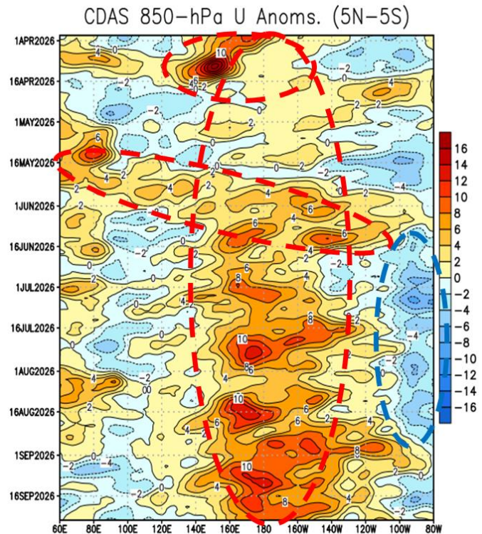
Figura 6 – Anomalías de viento zonal promediado en la región 5°S-5°N del 01 de abril al 28 de septiembre de 2026 - Fuente: Climate Prediction Center (CPC)-NOAA
