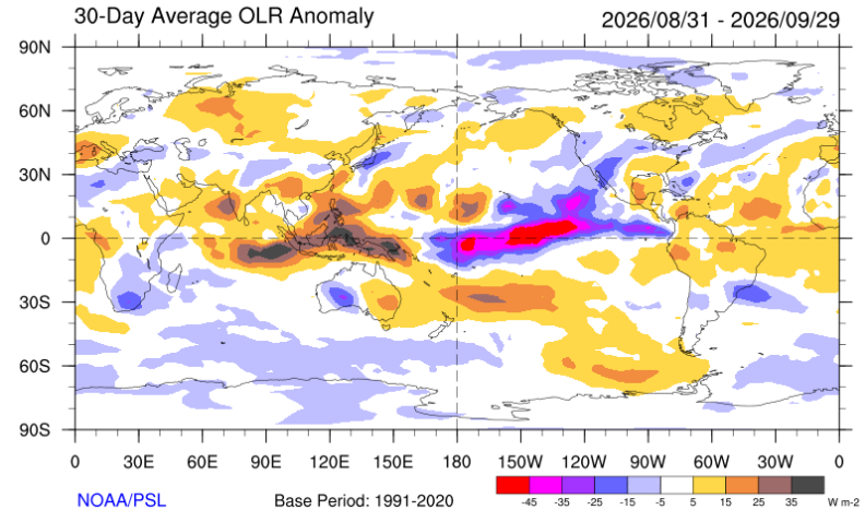
Figura 8 – Promedio de anomalías de radiación de onda larga saliente (OLR) del 31 de agosto al 29 de septiembre de 2026 - Fuente: NOAA-CIRES/CDC
