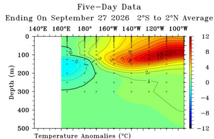
Figura 4 – Corte profundidad vs. longitud de la anomalía de temperatura del agua del mar en el Pacífico ecuatorial, correspondiente al promedio mensual de septiembre (izquierda) y pentádico que termina el 27 de septiembre (derecha). Fuente: Pacific Maritime Environmental Laboratory (PMEL)-NOAA
