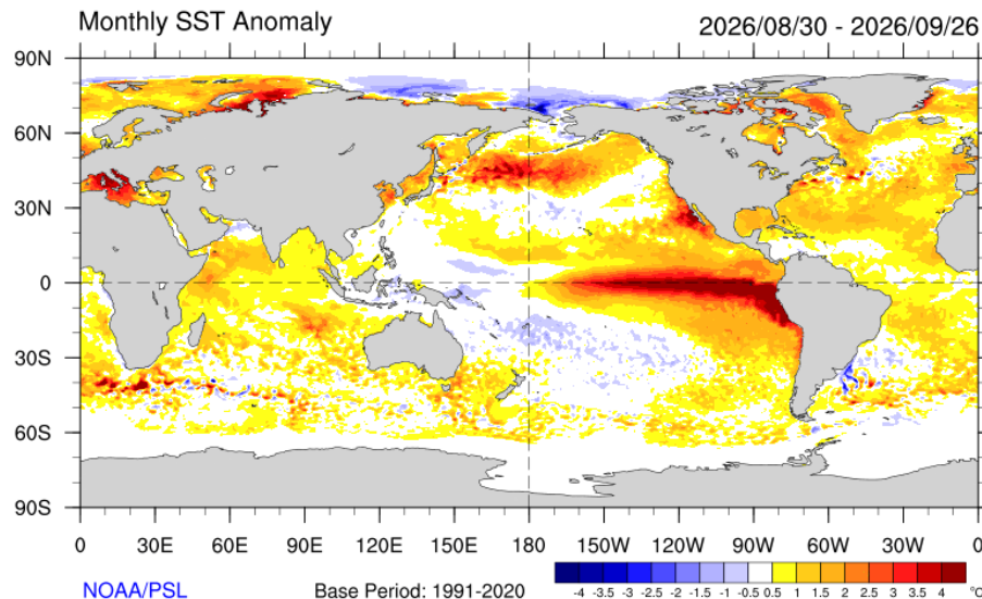
Figura 1: Anomalías de la temperatura superficial del mar del 30 d agosto al 26 de septiembre de 2026. Período de referencia 1991-2020 Fuente: NOAA-NCEP/CPC
